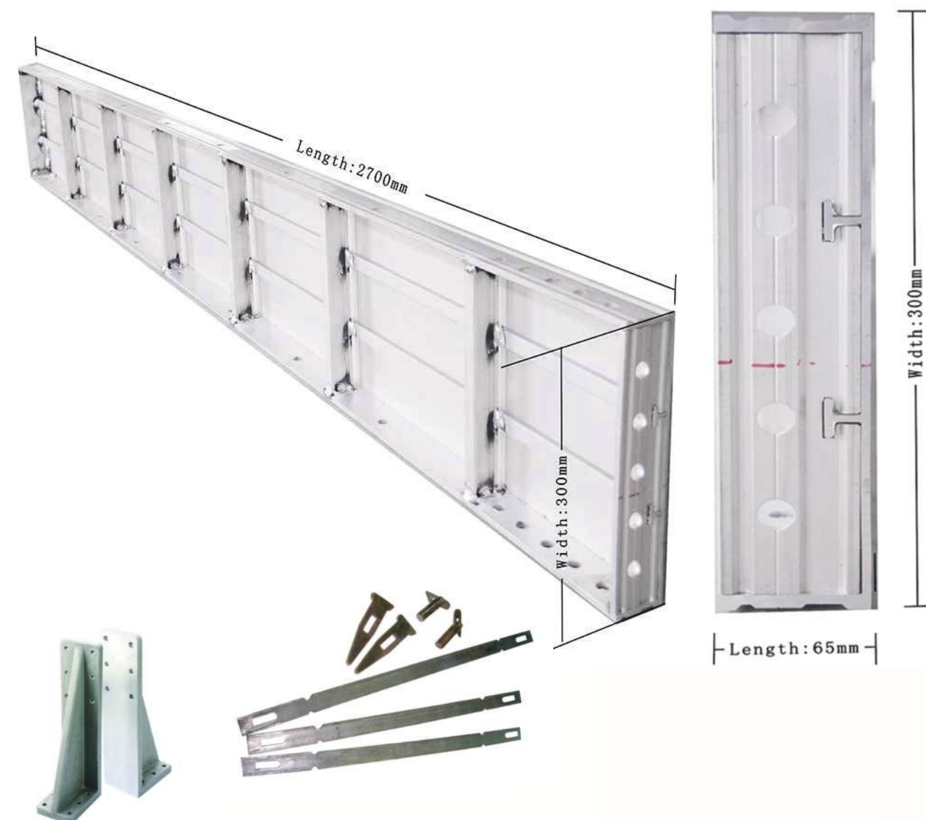
HỆ COPPHA NHÔM VÀ PHỤ KIỆN ALUMINUM COPPER SYSTEM AND ACCESSORIES
